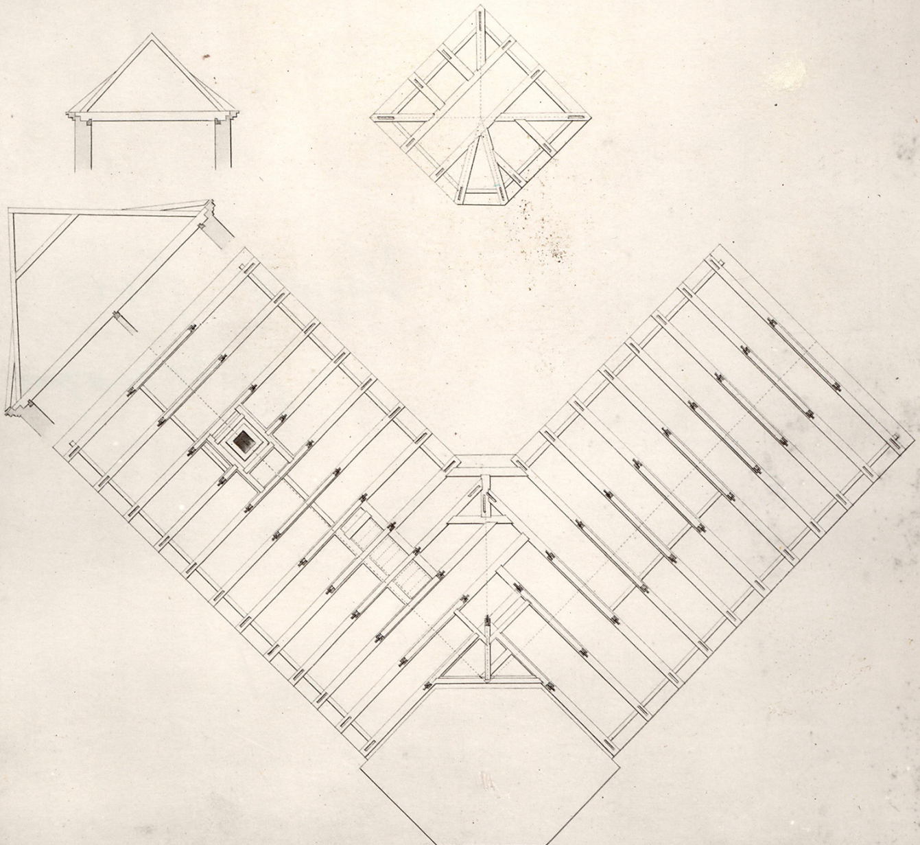
Plan af Bjelkelagene med Profiler.
